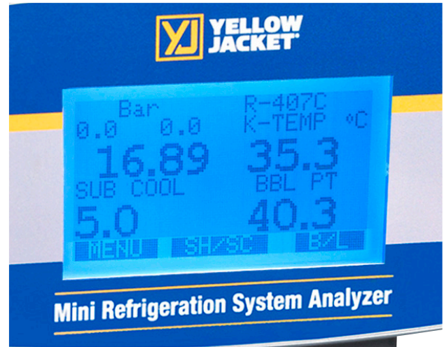
bar - Subcool
