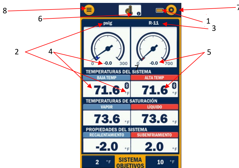
Figura 18: Diagrama del modo presión/temperatura
