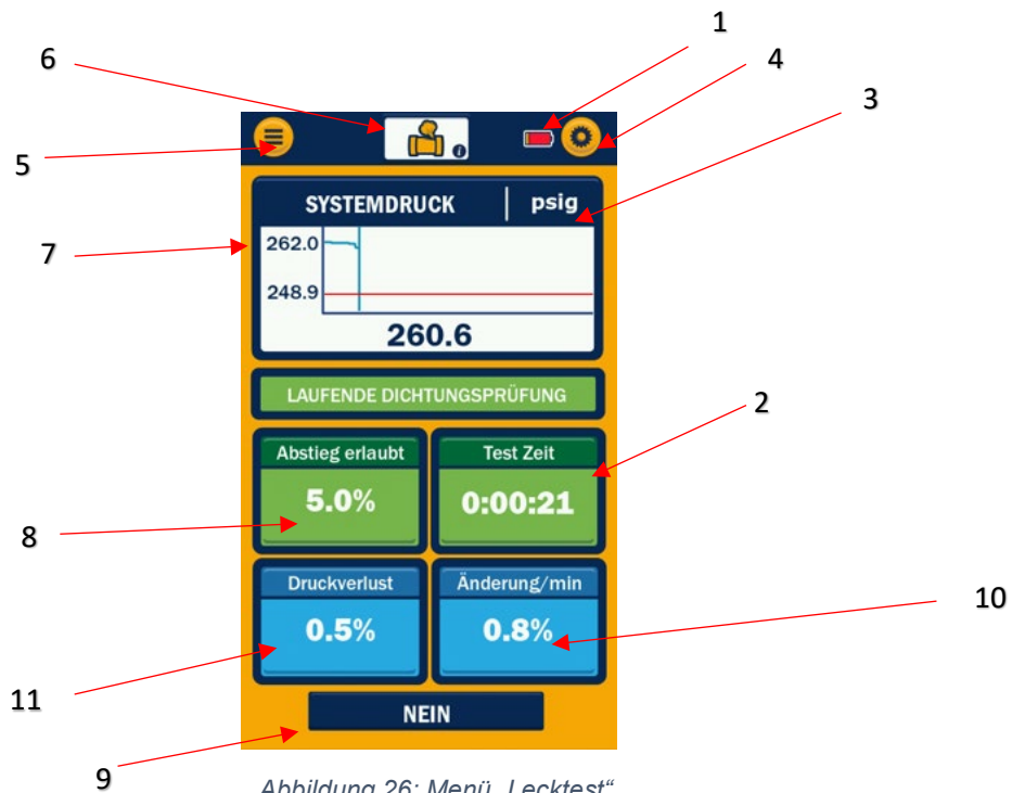
Abbildung 26: Menü „Lecktest“.
